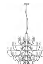
SM325S2 Φ1000×H880(MAX H2000)
